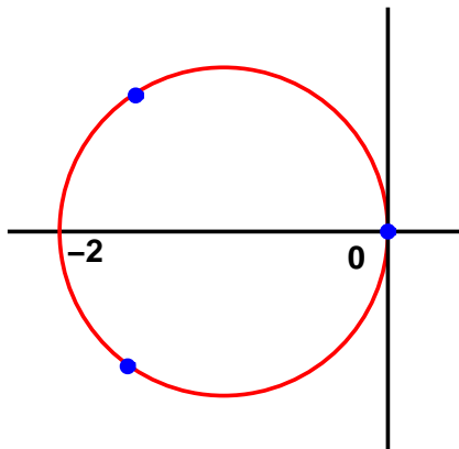
FIG. VII.4. Eigenvalues of S
