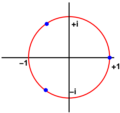
FIG. VII.4. Eigenvalues of S
