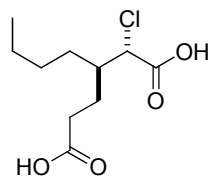
(2S,3R)-3-butyl-2-chlorohexanedioic acid
