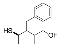
(4R)-3-benzyl-4-mercapto-2-methylpentan-1-ol
