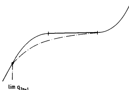
Fig. 2.2. The construction of Lemma 2.1.
